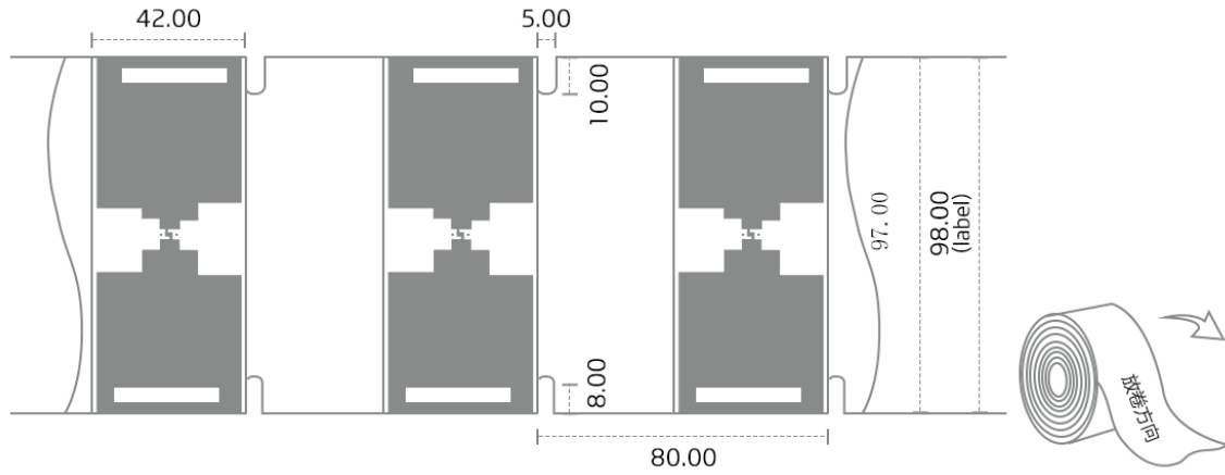
标签结构图
