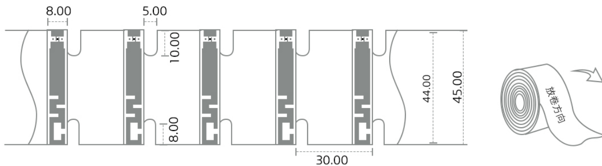
标签结构图
